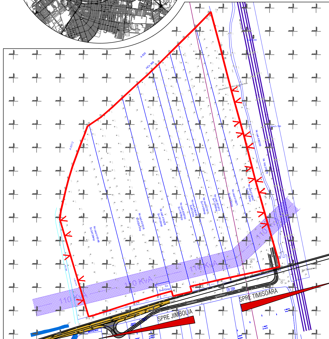
INCADRARE - PLAN TOPOGRAFIC
